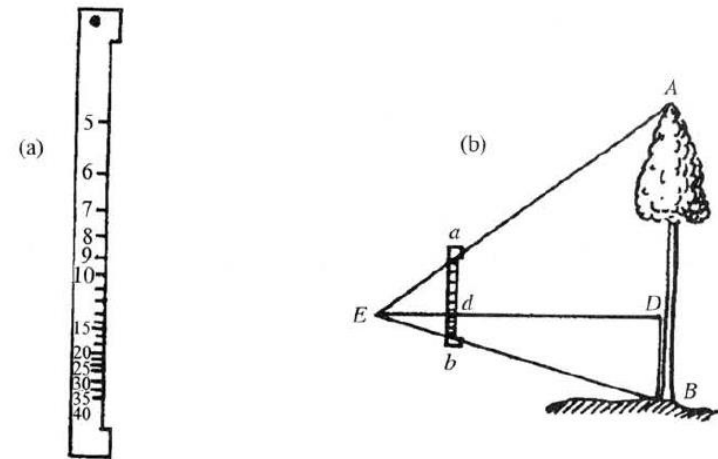
Christen測高儀及其使用方法之圖解
